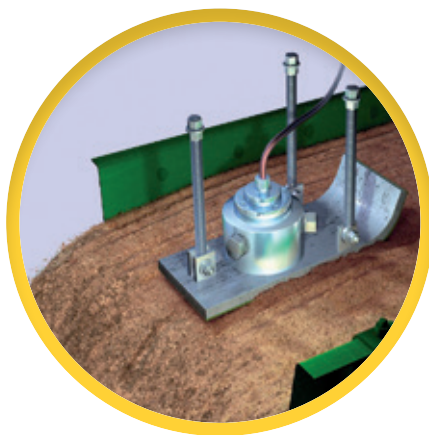
Op een doseertransportband of op een trilogoot.
