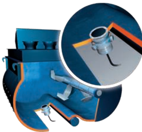
In de kuip van een horizontale menger.
