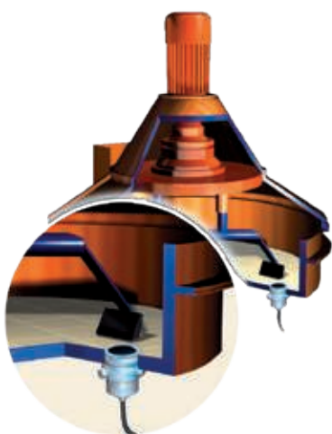
Op de bodem van een planetaire menger.
