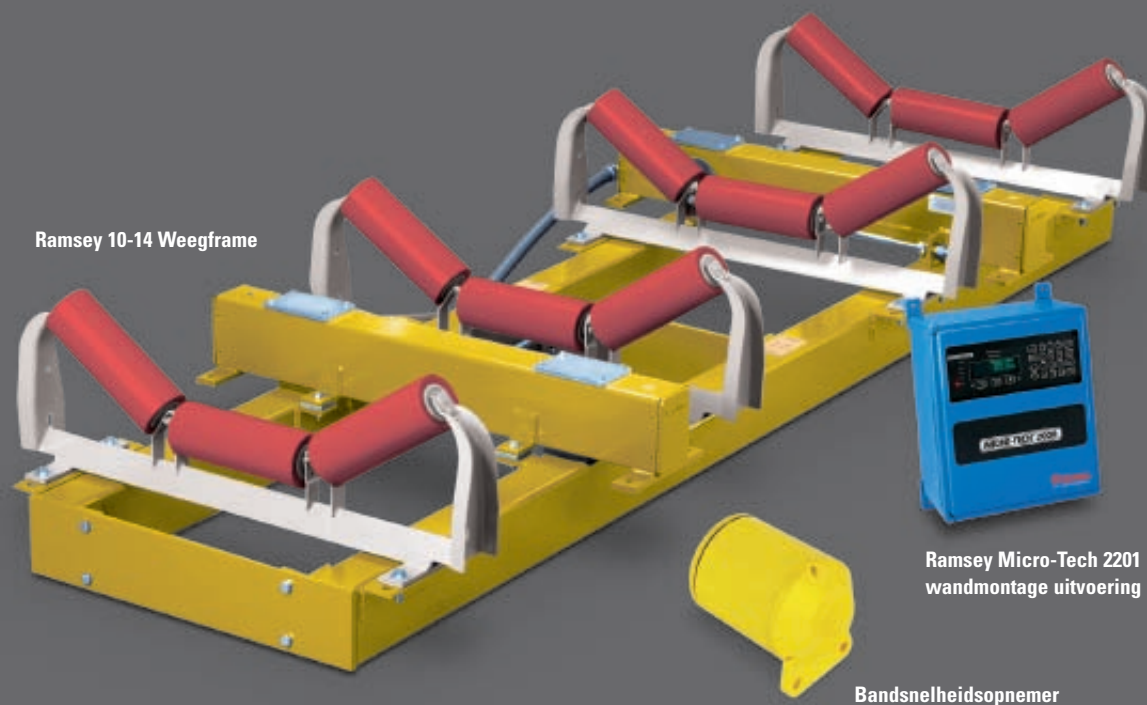
Bandsnelheidsopnemer
