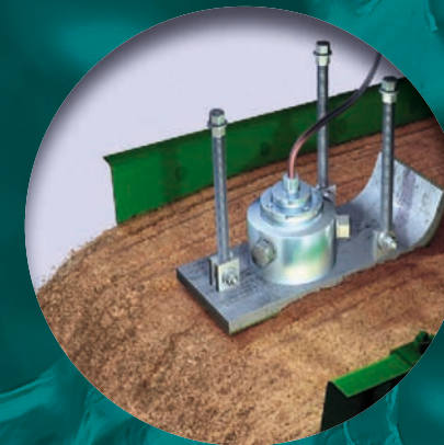
Sur la bande de dosage ou une goulotte de vibration.
