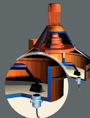
Installation dans le fond mélangeur d'un mélangeur de planète.
