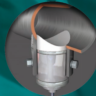
Montage dans un tube.
