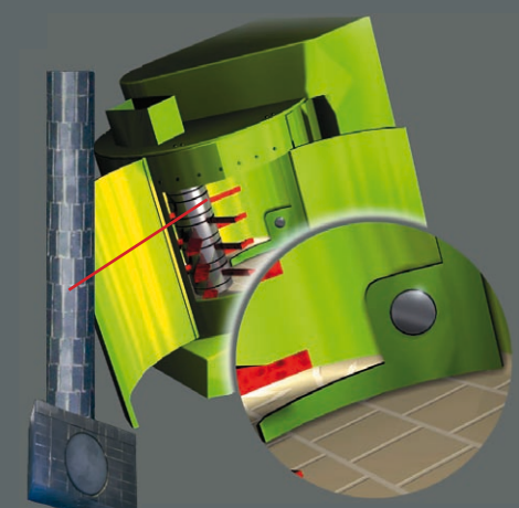
Installation dans la bande latérale d'un mélangeur intensif.
